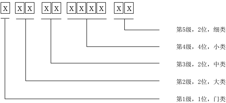
图 1 代码结构图
